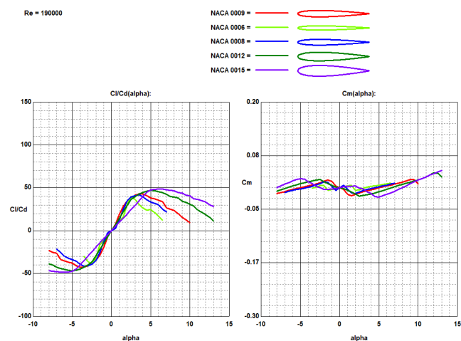
图 10: 升阻比, 俯仰力矩系数随攻角的变化
