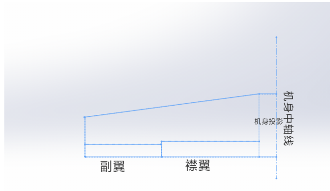
图 4: 襟翼副翼布置图
